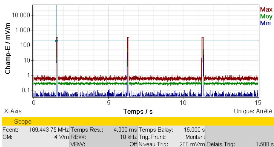
Figure 10 : analyse temporelle d'une trame test déclenchée par le PDA de maintenance et composée de 3 impulsions de 120 ms
